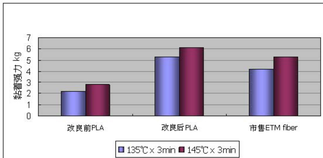
<图一> PLA 热黏着纤维与天然纤维之黏着强力
