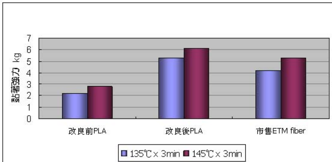
<圖一> PLA 熱黏著纖維與天然纖維之黏著強力
